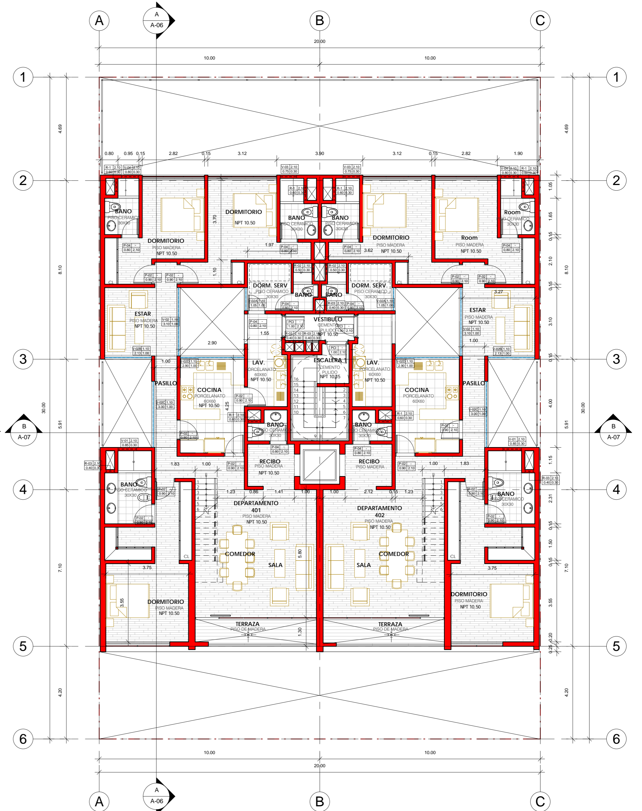
2 4° PISO 1 : 100
