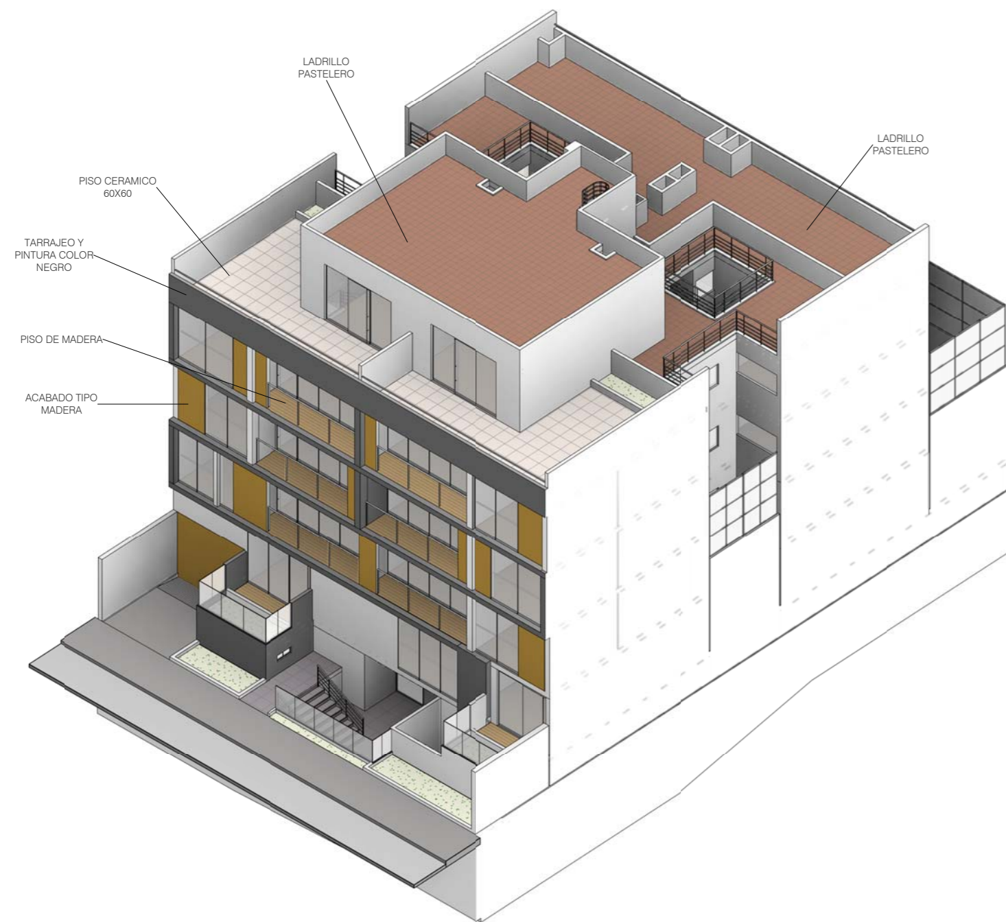
1 ACABADOS EXTERIORES
