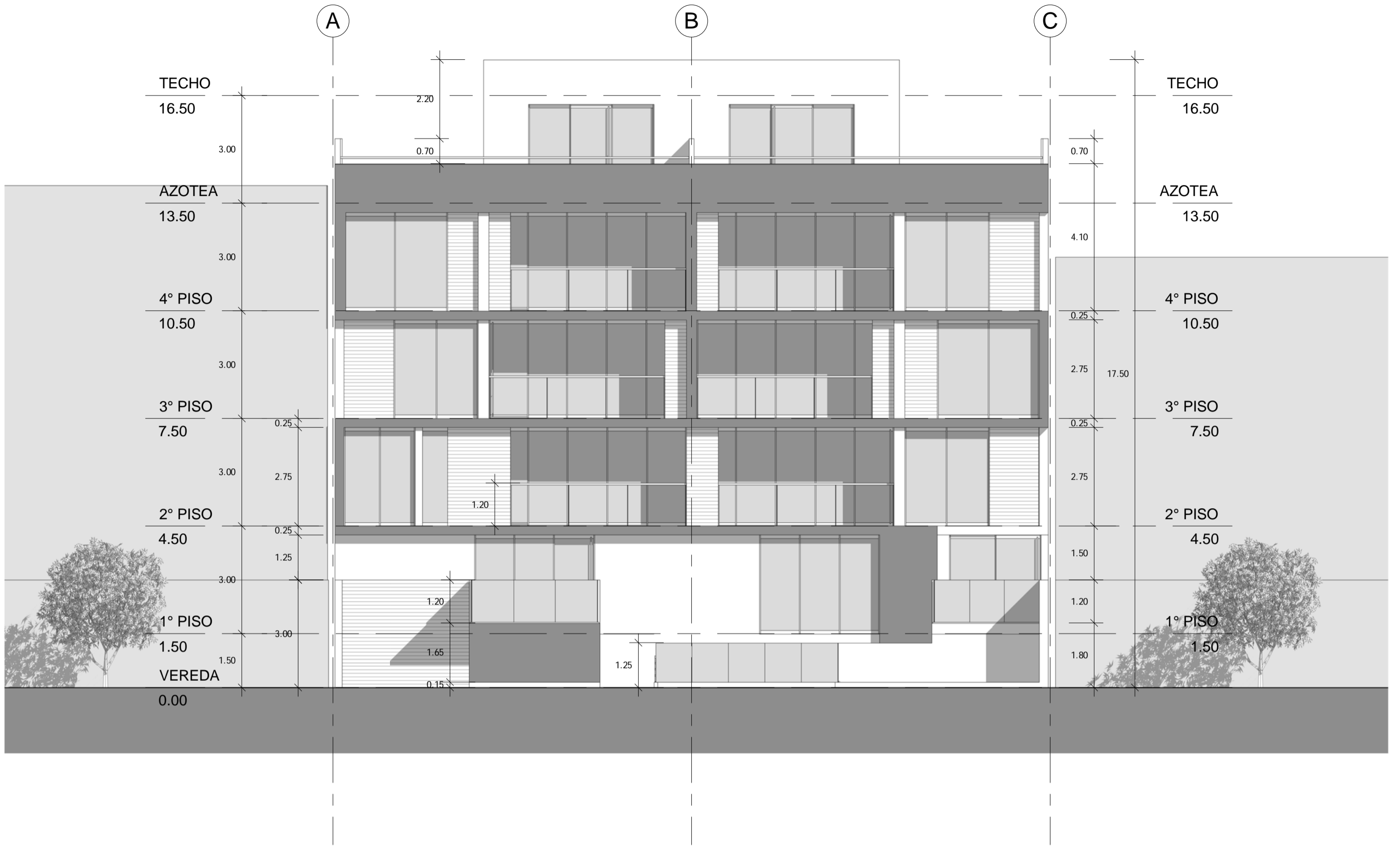
1 ELEVACION PRINCIPAL 1 : 100
