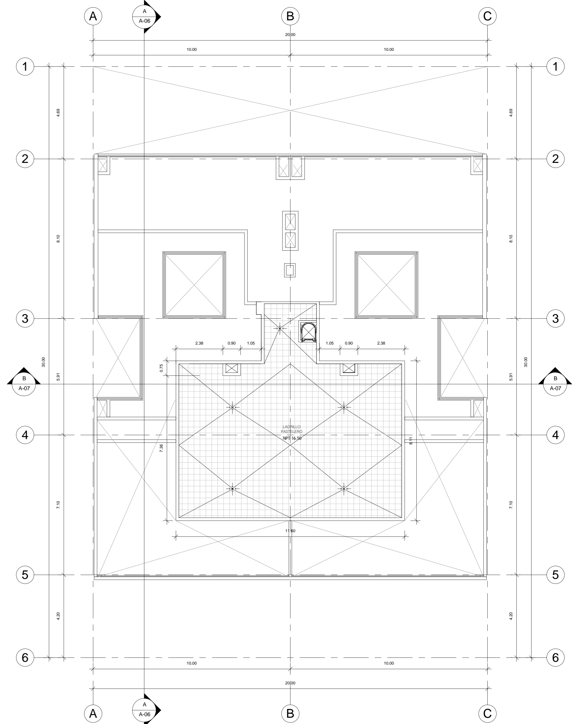
2 TECHO 1 : 100
