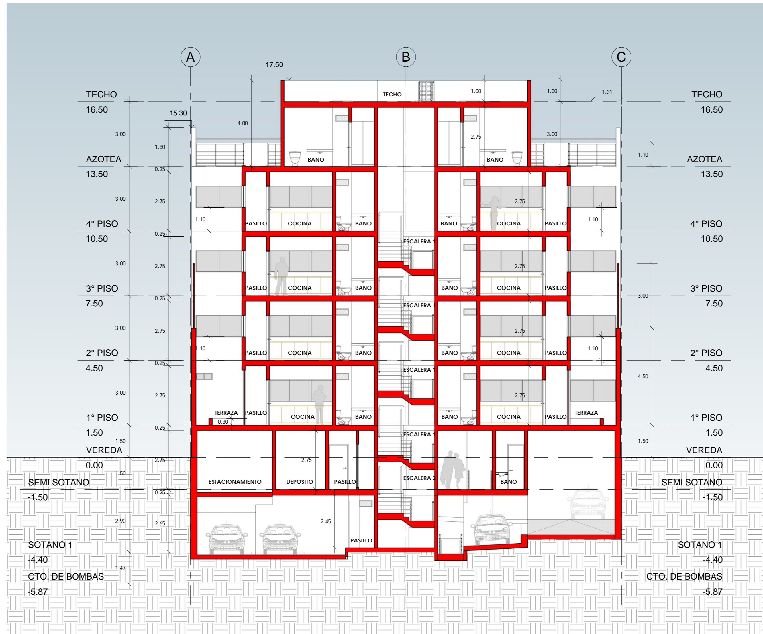
B CORTE B 1 : 100
