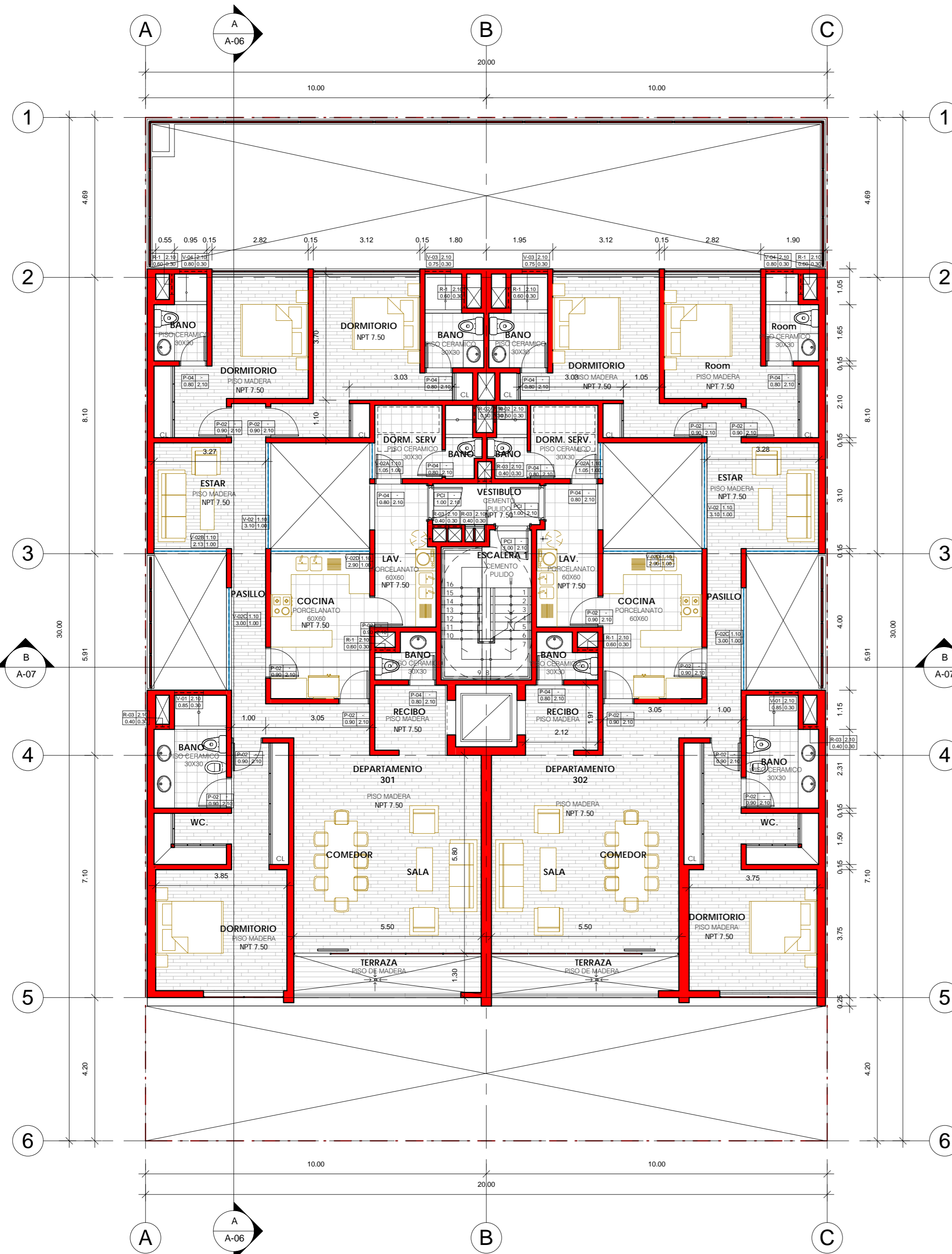
1 3° PISO 1 : 100
