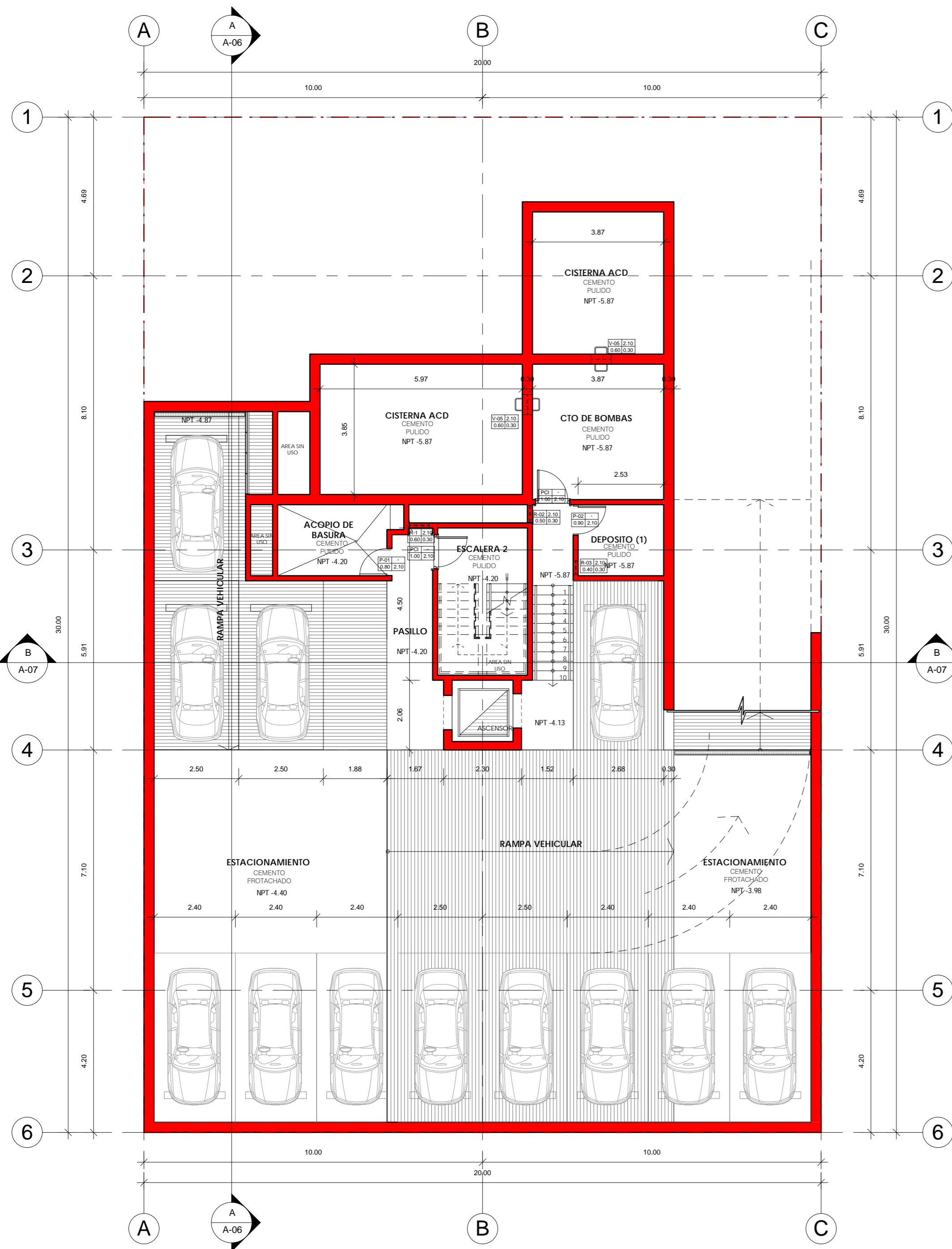
1 SOTANO 1 1 : 100
