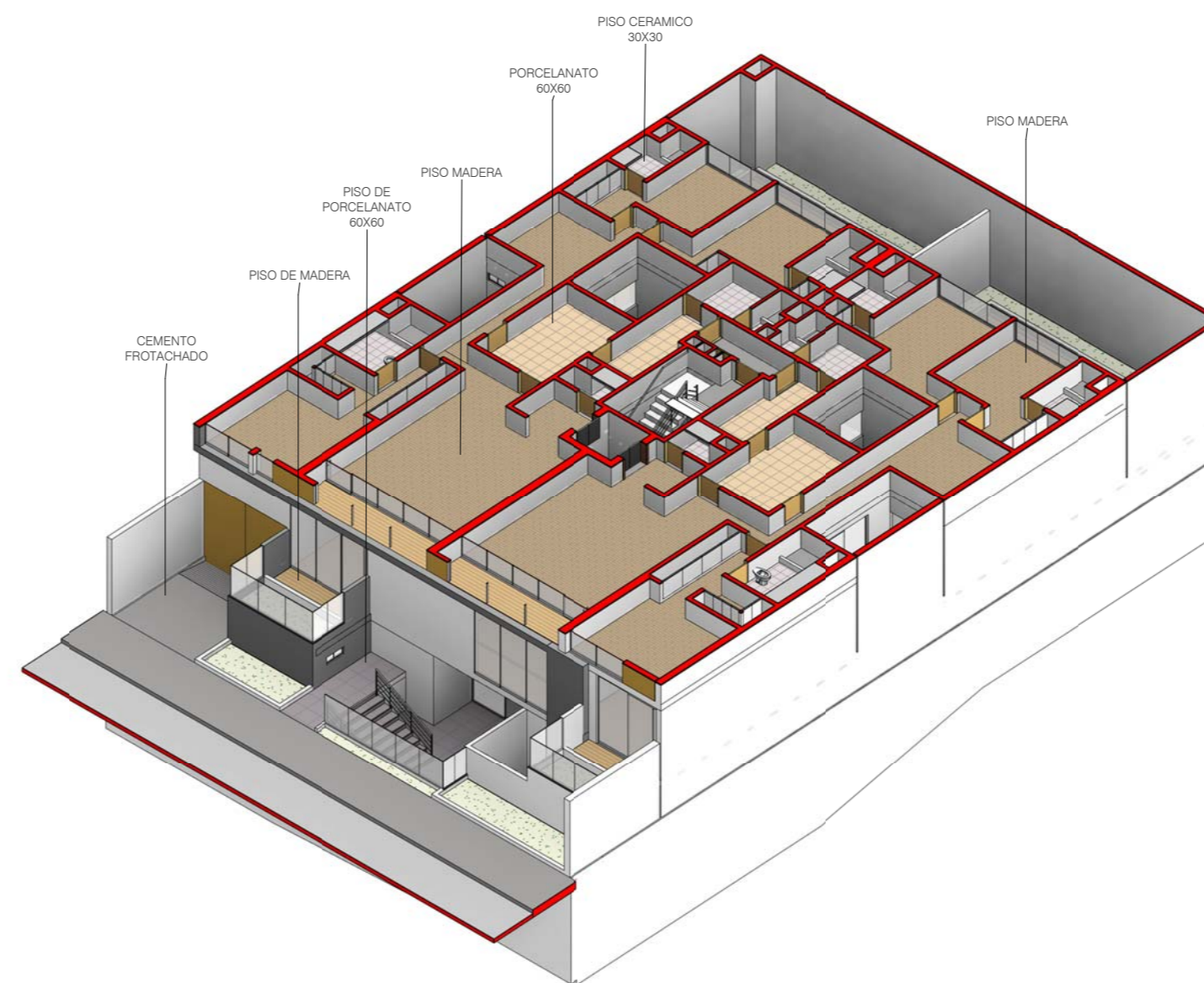
2 ACABADOS PISOS
