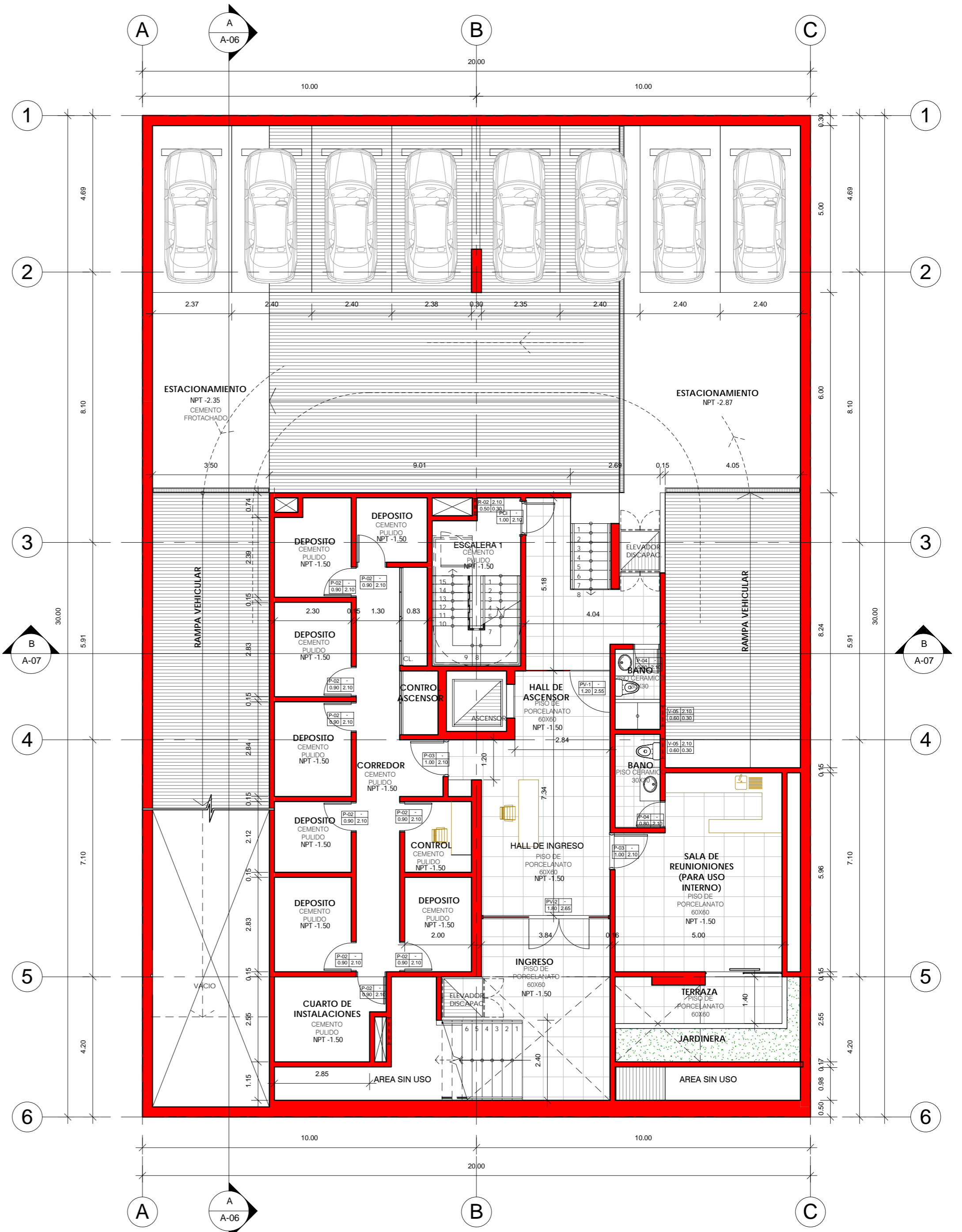
2 SEMI SOTANO 1 : 100
