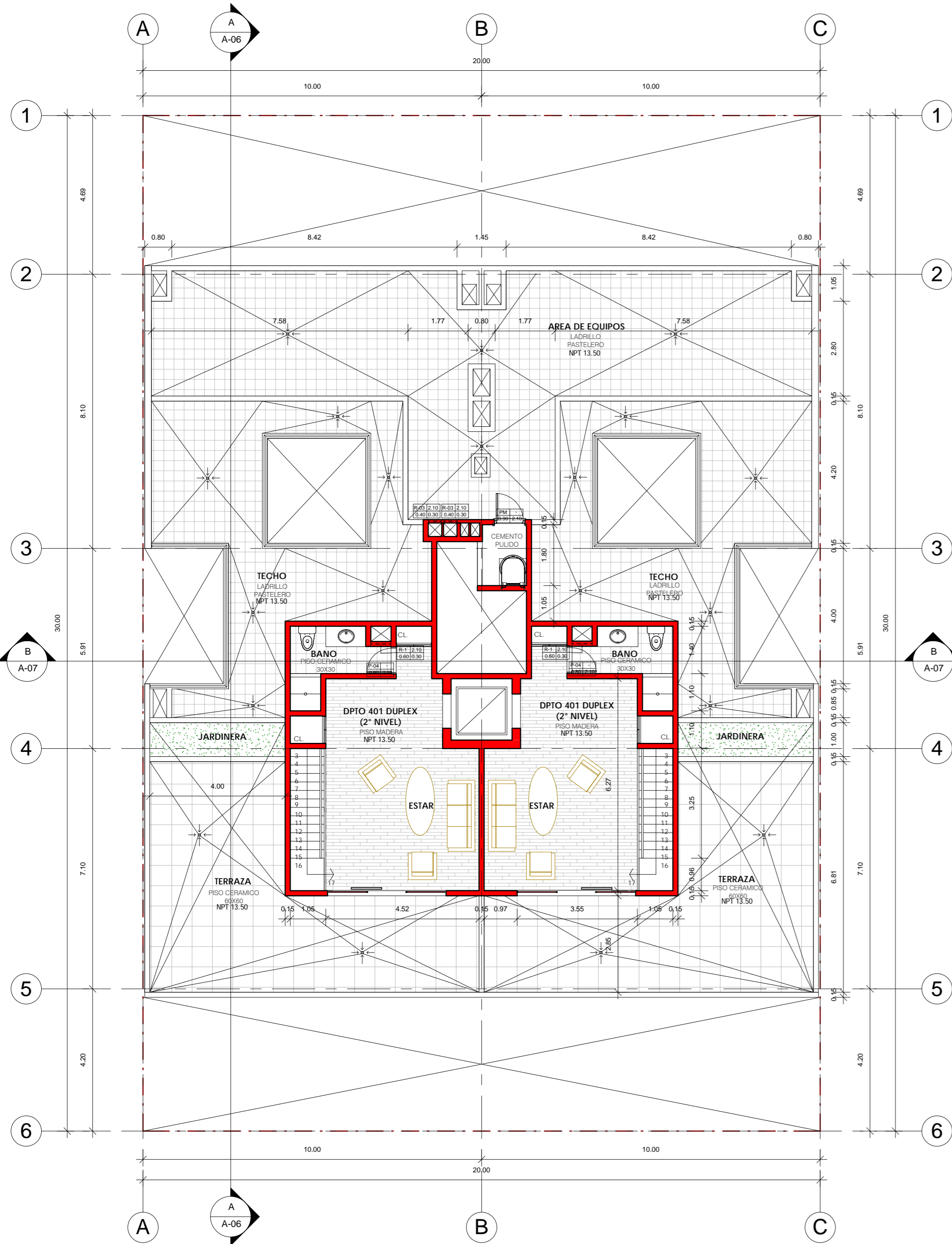
1 AZOTEA 1 : 100
